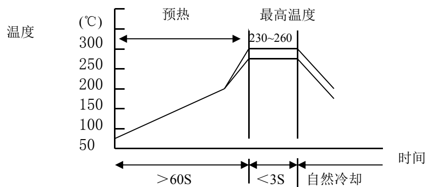
(b) 波峰焊接温度曲线图
