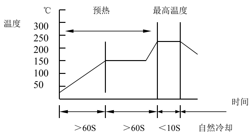
(a) 回流焊接温度曲线图
