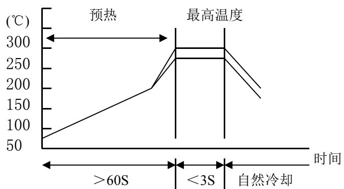
(c) 手工焊接温度曲线图
