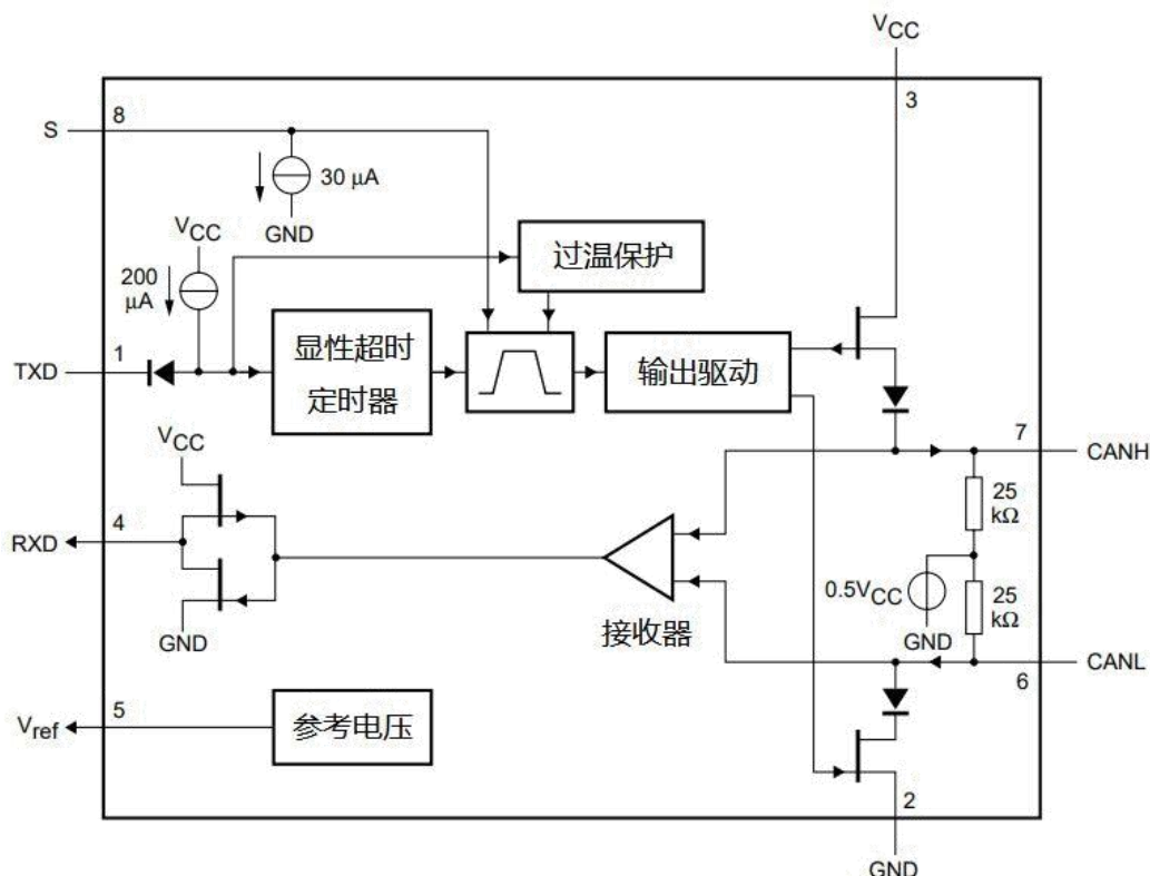
图 1: TJA1050T 逻辑图
