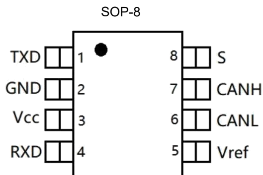
图 2: TJA1050T 引脚图
