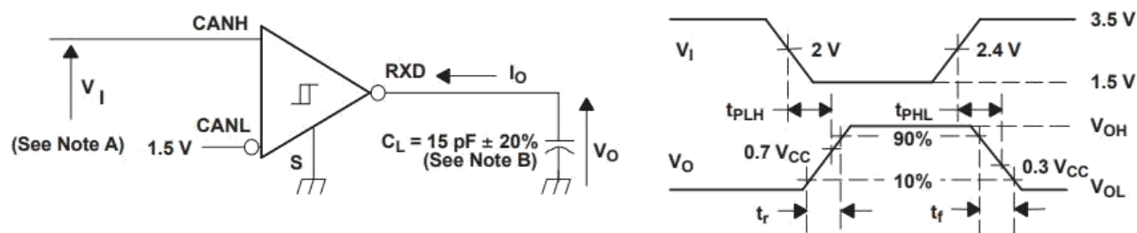
图 8：接收器测试电路和电压波形
