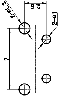
PCB线路板安装图(±0.1)
