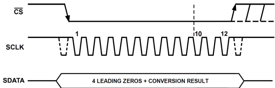
时序图
