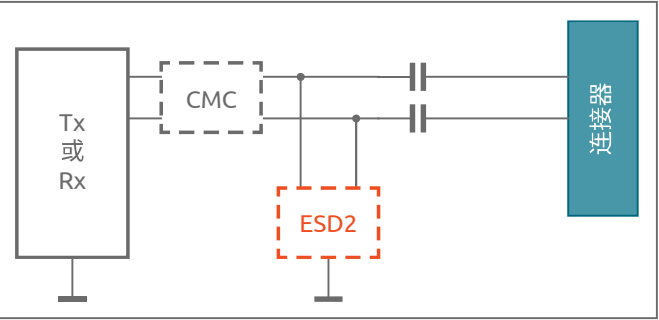
方案2：在直流电容后面
