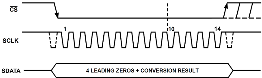
时序图
