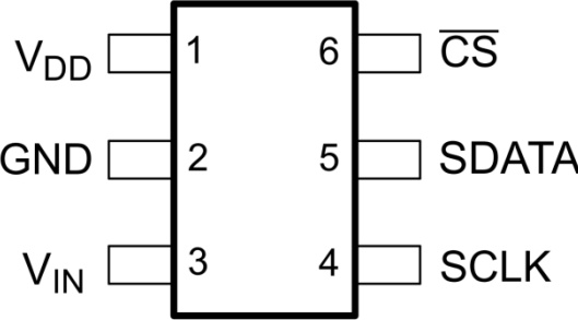
引脚图
