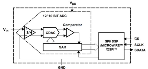
原理图
