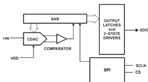
原理图
