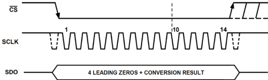
时序图
