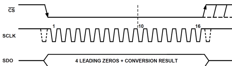
时序图
