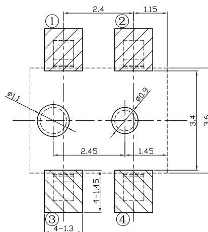
安装位置图
