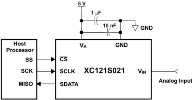
电路连接图
