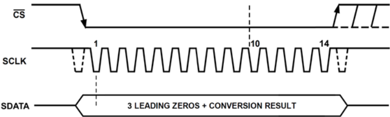
时序图
