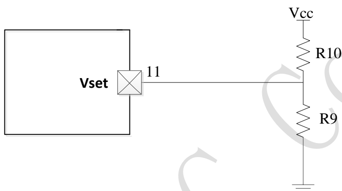
图 8 Vset 电池电压配置电路
