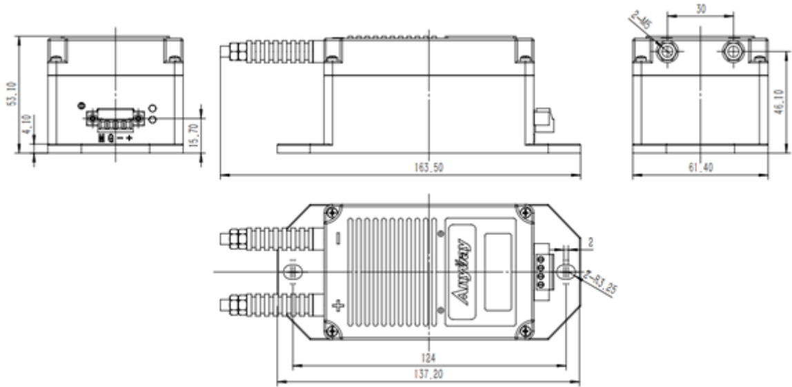
图 1 外形尺寸图
