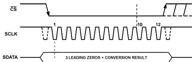
时序图
