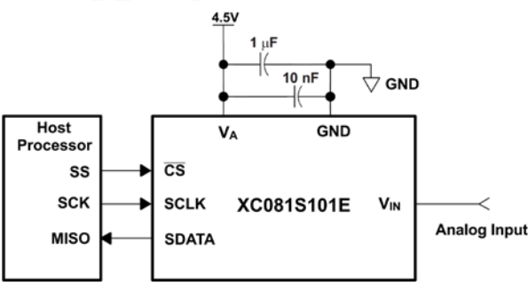
电路连接图
