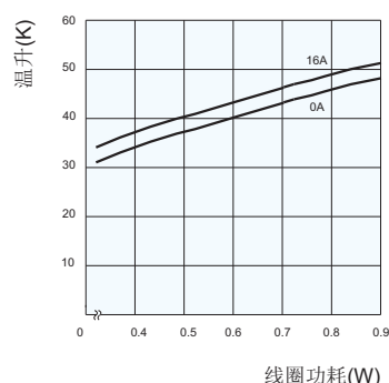
线圈温升
