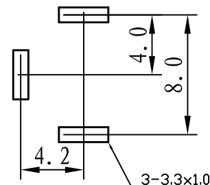
线路板安装尺寸示意图
