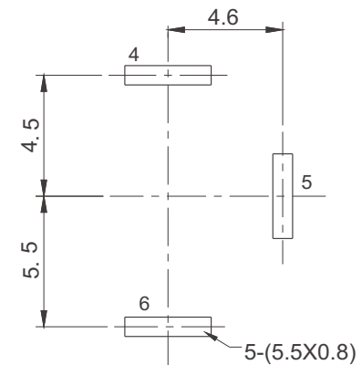
线路板印制示意图
