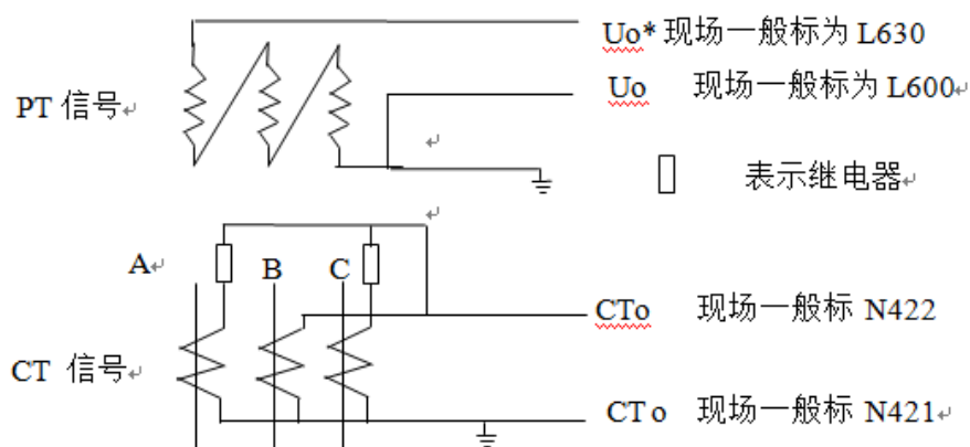
图 (9.1) 现场 PT、CT 信号箱
