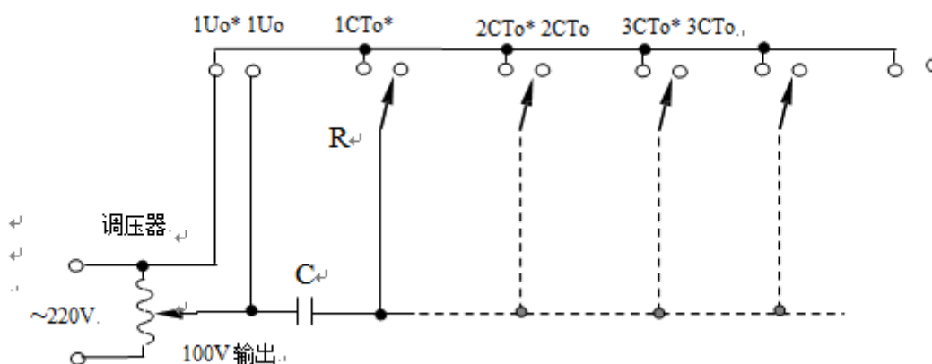
9.3 模拟试验图
