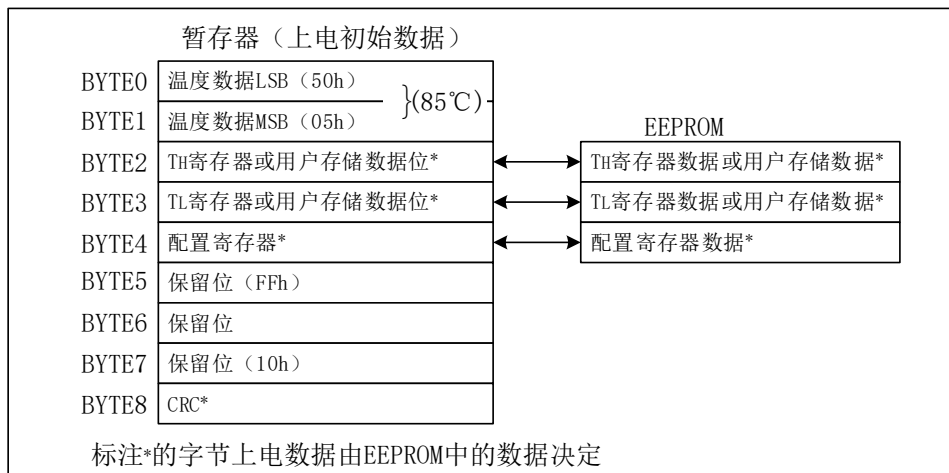
图 2-5 DS18B20-TD存储器映射
