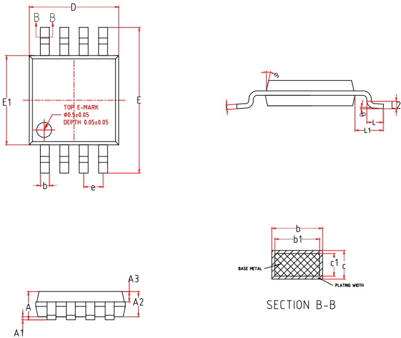
MSOP8 外形图
