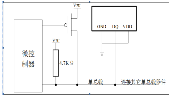
图 2-2 在温度转换期间提供寄生供电
