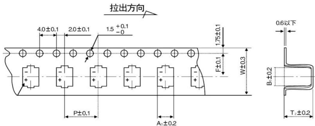
Fig.1 (Ø4 ~ Ø10)
