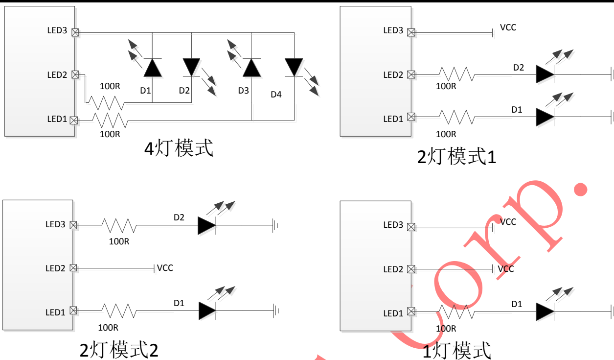
图 6 4、2、1LED 连接方式
