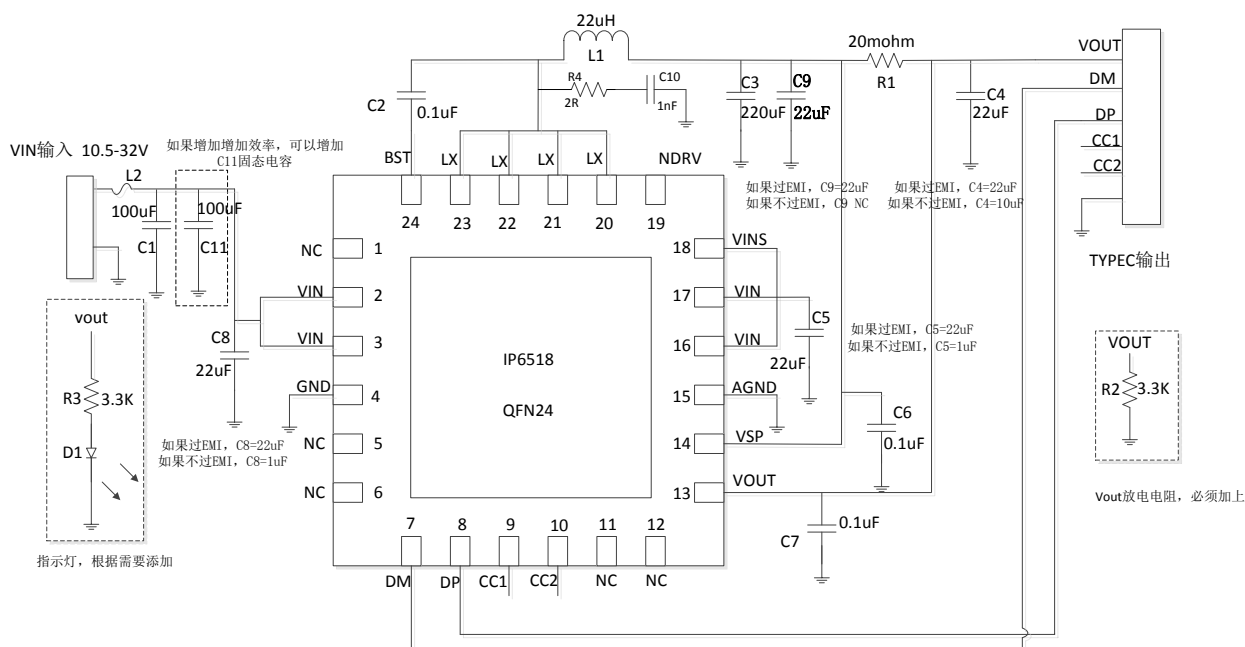
图 6 TYPE-C 口 PD 快充输出应用原理图
