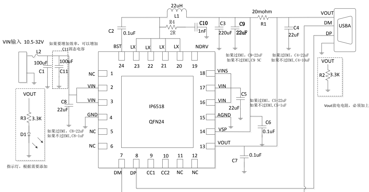
图 5 USB 口输出应用原理图
