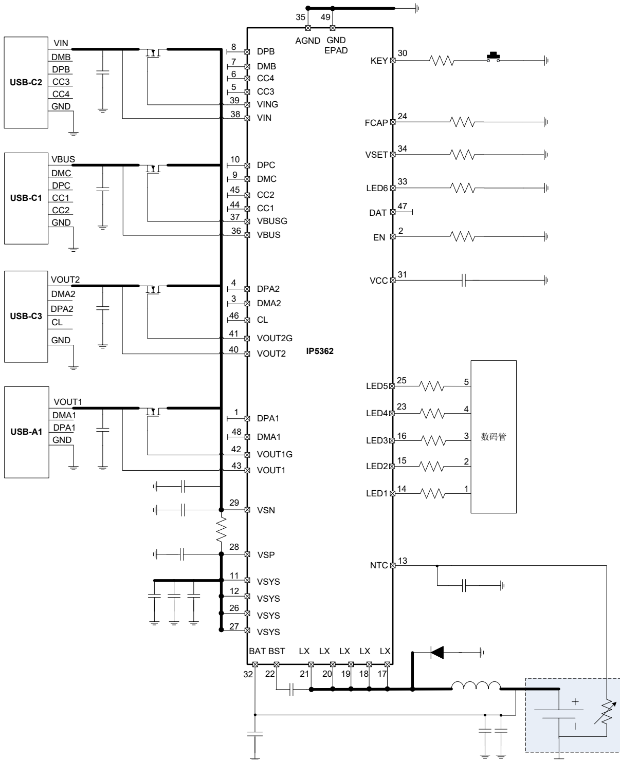
图 1 简化应用原理图
