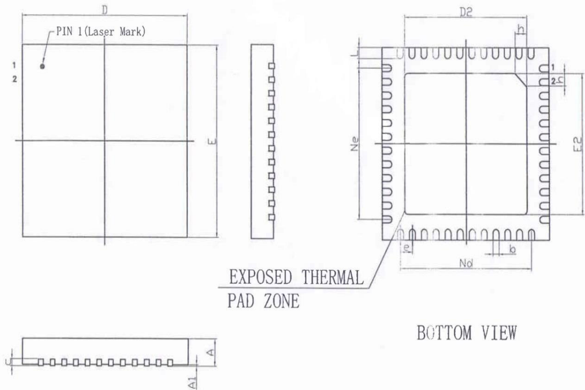
图 36 IP5362 封装尺寸图
