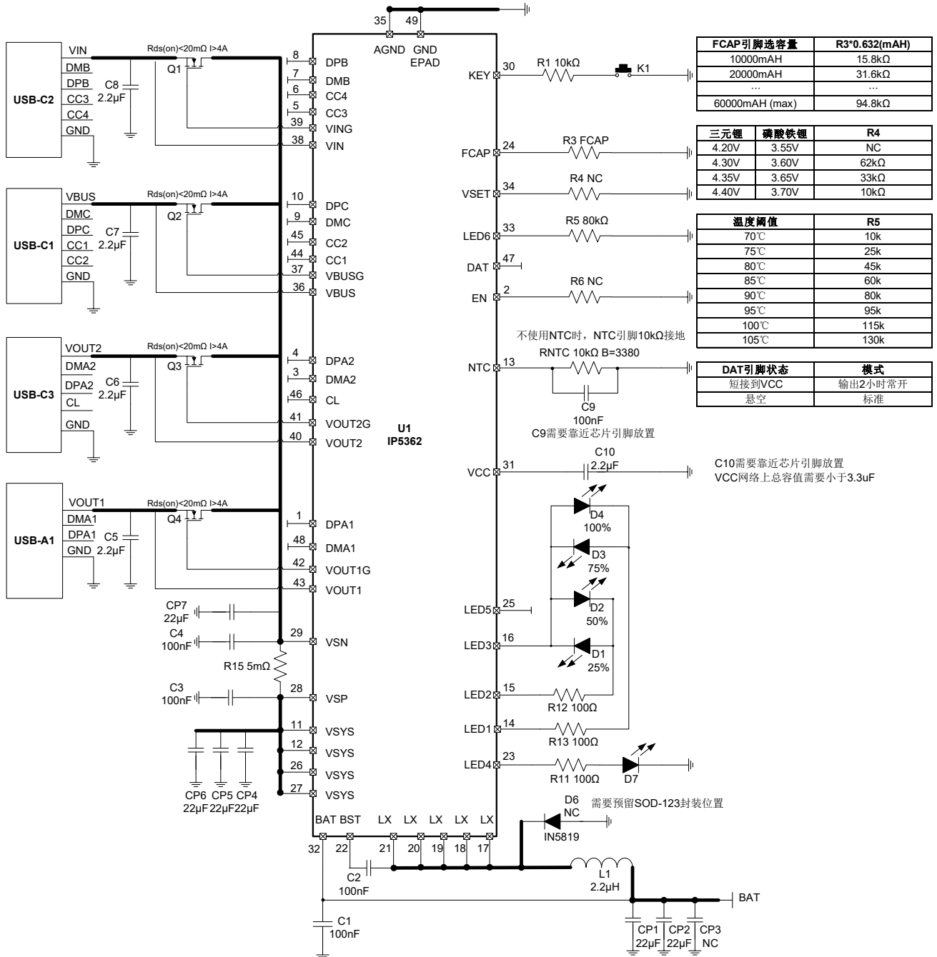
图 33 IP5362_ACCCO_LBZ 系列典型应用原理图
