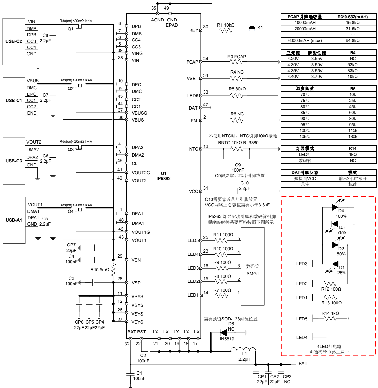
图 34 IP5362_AACC_BZ 系列典型应用原理图
