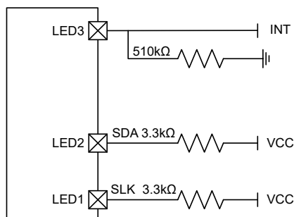
图 26 I2C 应用电路图
