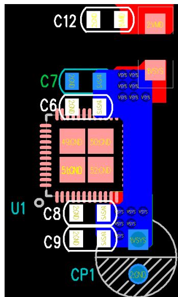
图 28 VSYS 电容
