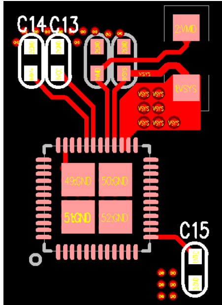
图 29 BAT/VCC/VDD/NTC1 电容
