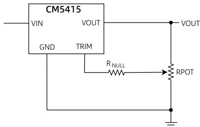
图 12 微调输出功能
