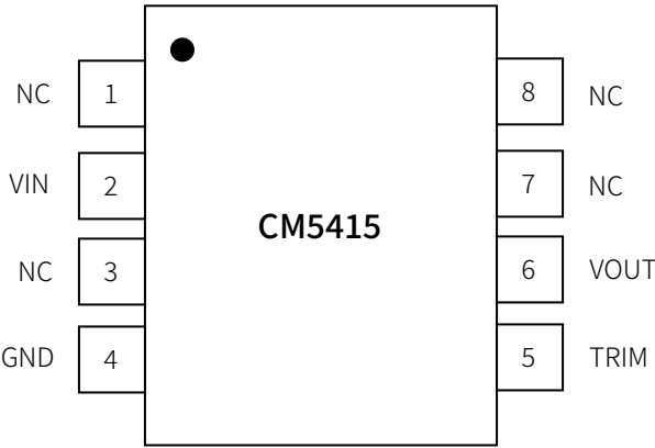
图 1 管脚示意图（顶视图）
