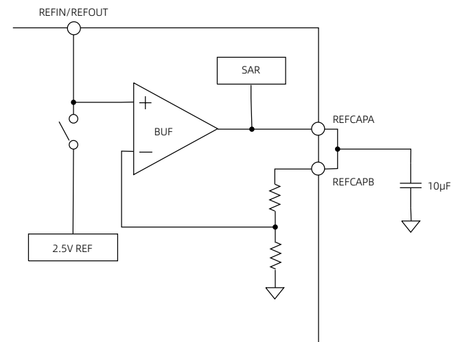
图 45 基准电压电路
