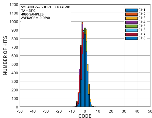
图 25 零输入直方图, \pm 10V 单端输入
