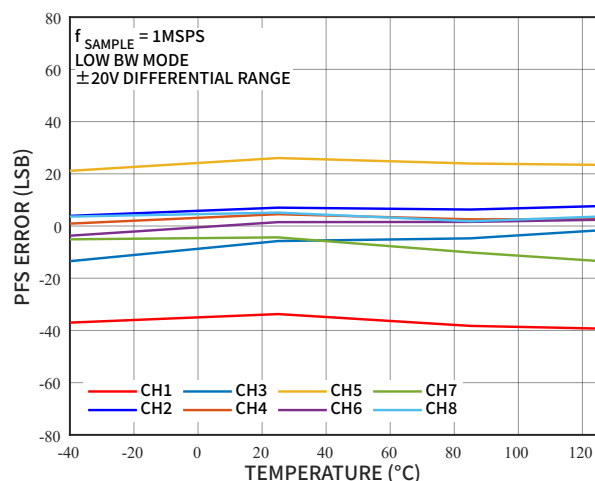
图 21 PFS 误差的温度特性, \pm 20V 差分输入
