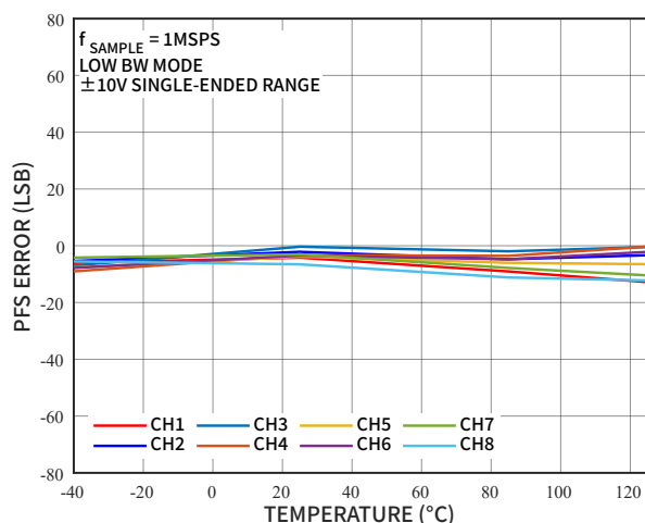
图 20 PFS 误差的温度特性, \pm 10V 单端输入
