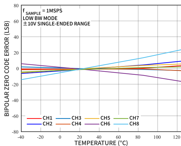
图 23 0 码误差的温度特性, \pm 10V 单端输入
