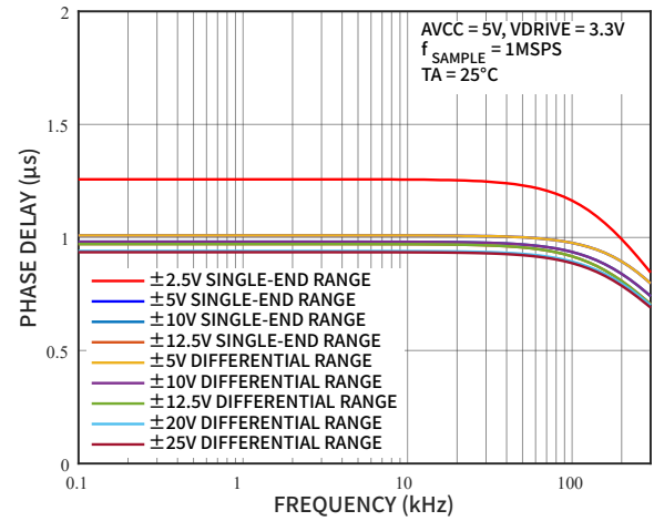
图 44 抗混叠滤波器相频特性，高带宽模式
