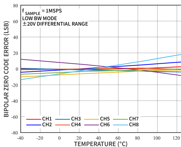
图 22 0 码误差的温度特性, \pm 20V 差分输入
