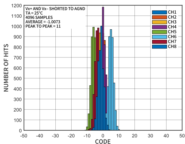
图 24 零输入直方图, \pm 20V 差分输入
