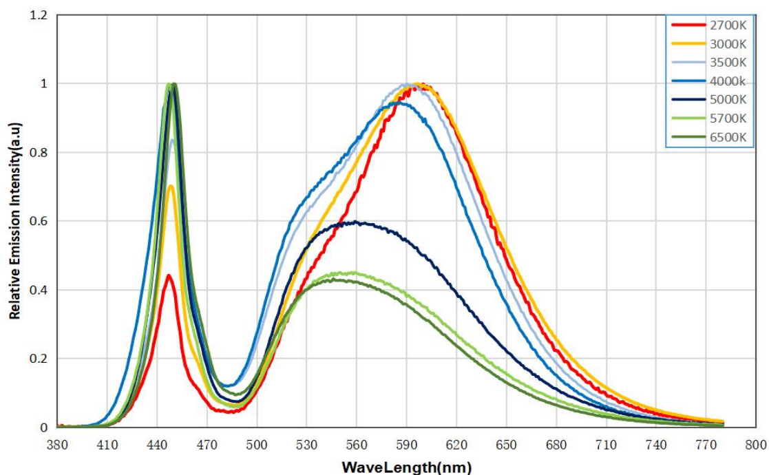
图2. 80显指光功率与光谱分布图
