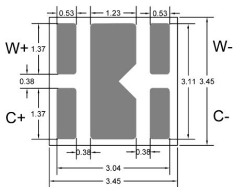
推荐 PCB 设计图
