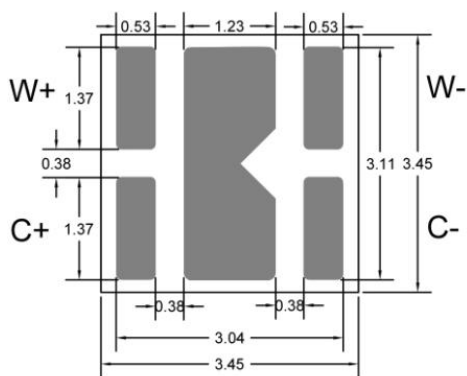
推荐焊盘设计图
