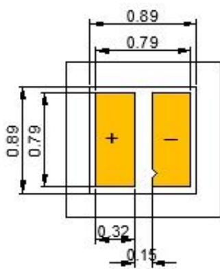
推荐焊盘设计图
