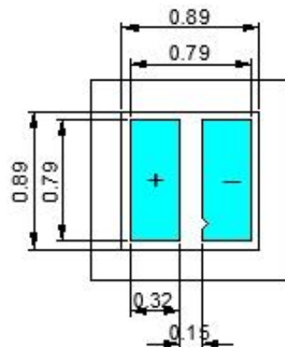
推荐 PCB 设计图
