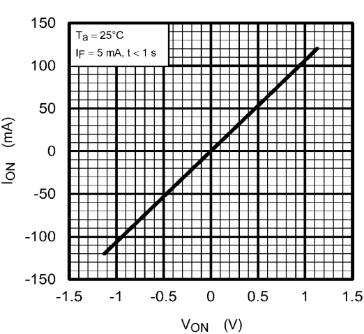
Fig. 12.4 I_{ON} - V_{ON}
