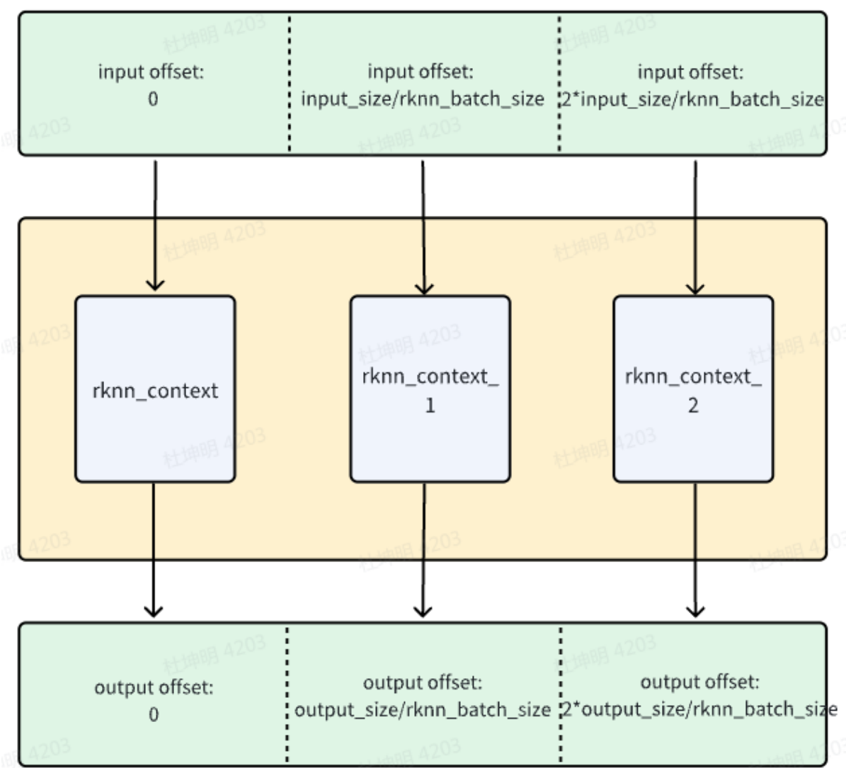
图5-15 多batch内部输入输出地址偏移图
