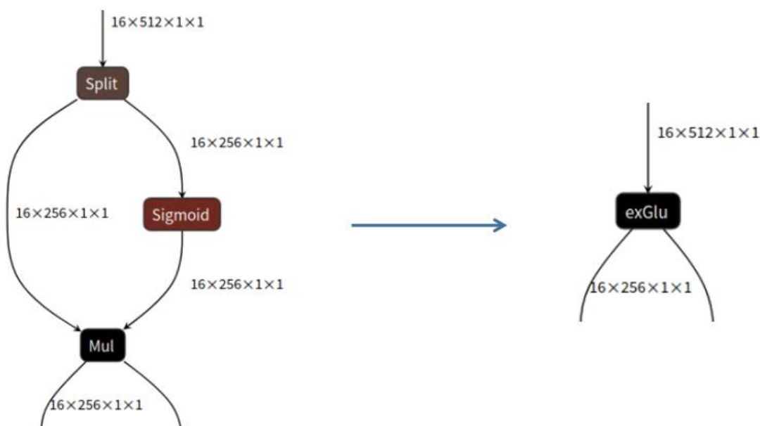
图8-13 Glu子图融合
