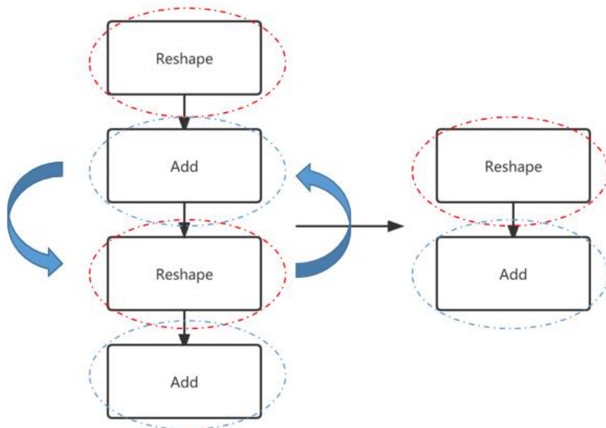
图8-10 同类项算子合并
