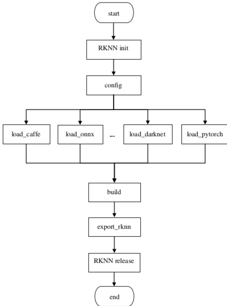
图3-1 模型转换流程图
