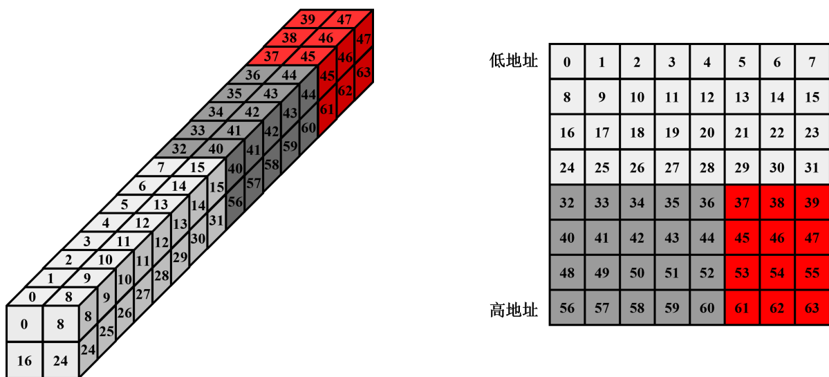
图5-2 NC1HWC2数据排布展开
