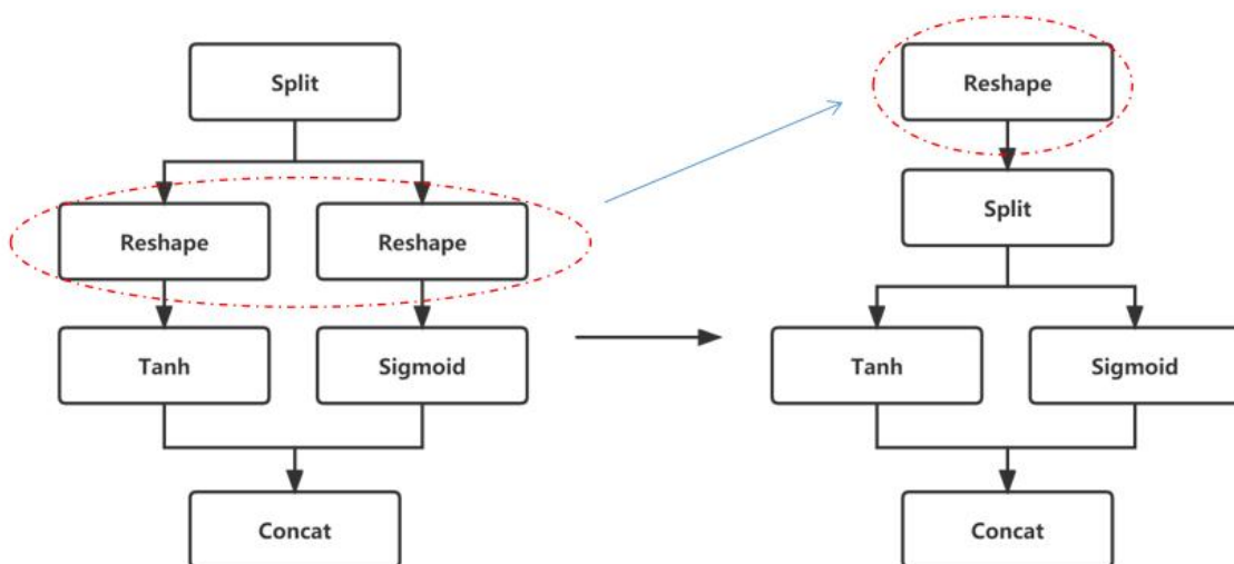
图8-11 重复性算子合并
