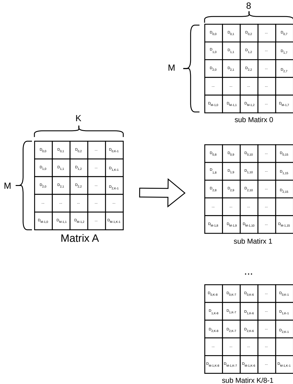
图3-8 int8类型矩阵A从[M,K]变换到[K/8,M,8]的元素对应关系图
