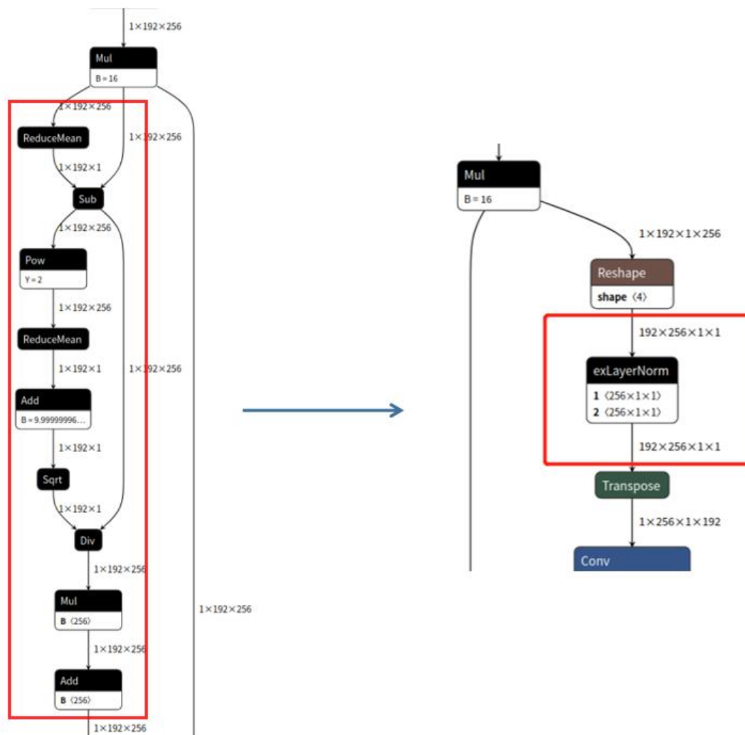
图8-14 LayerNorm子图融合
