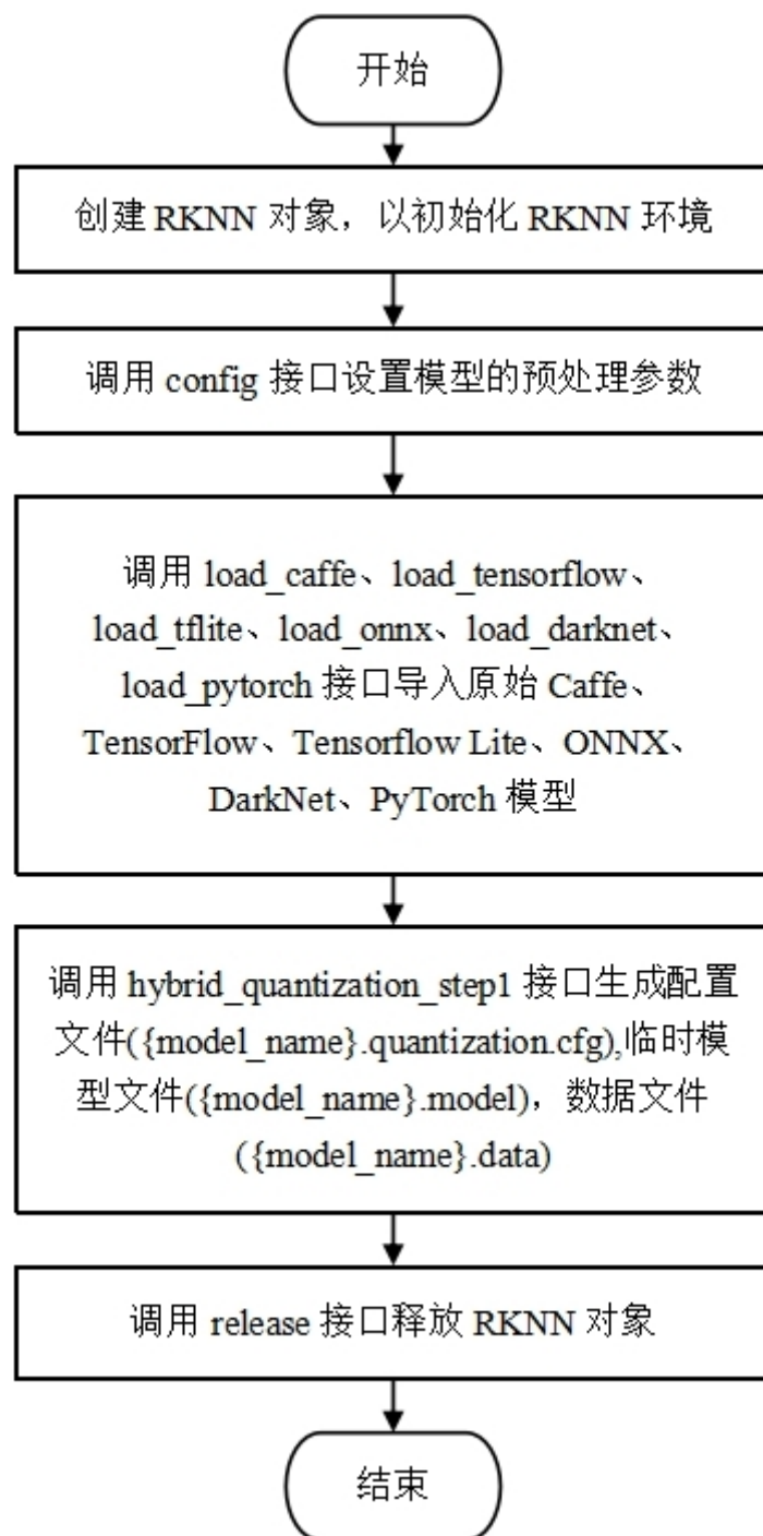
图6-3 混合量化第一步
