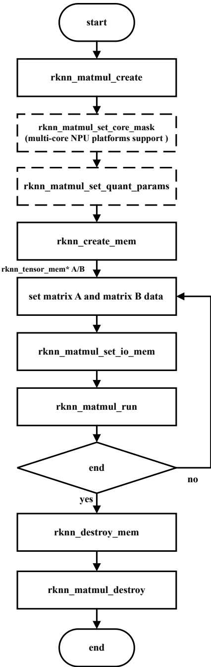
图3-6 Matmul API基础调用流程
