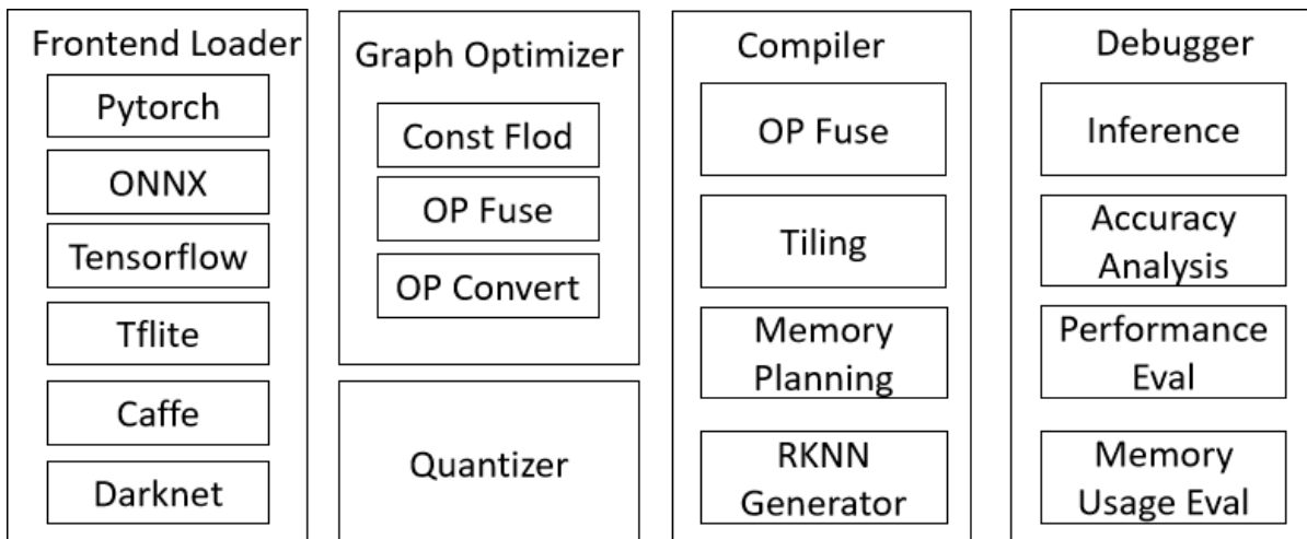
图 1-2 RKNN-Toolkit2 软件框图
