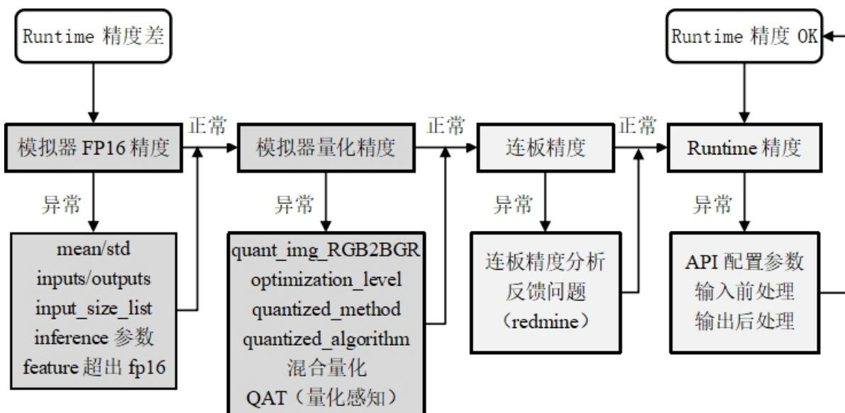
图7-1 精度排查步骤
