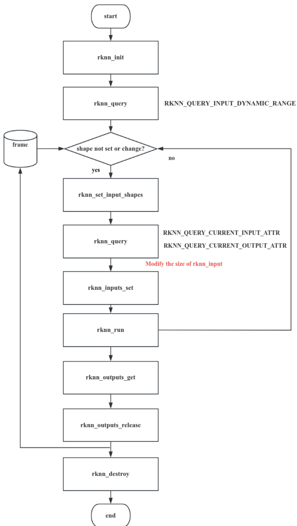
图5-10 动态shape输入接口的通用API调用流程
