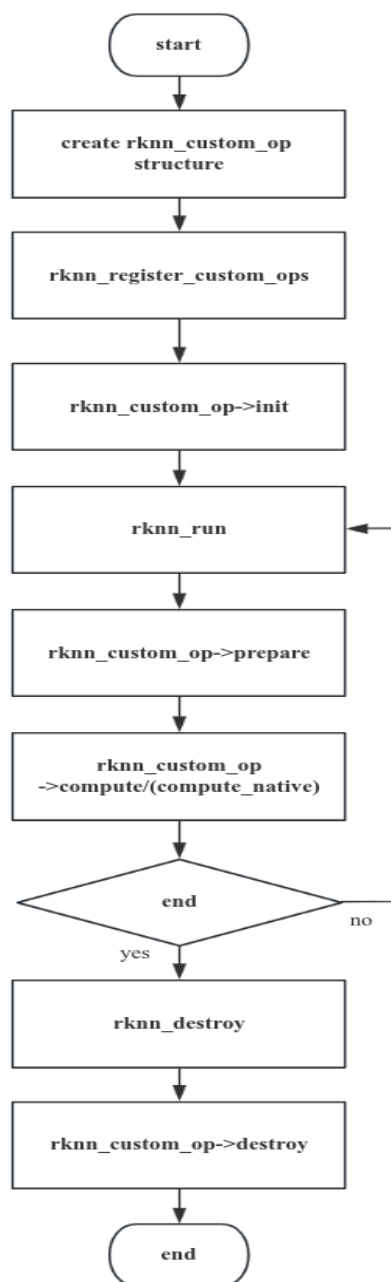
图5-13 注册自定义算子的C API调用流程
