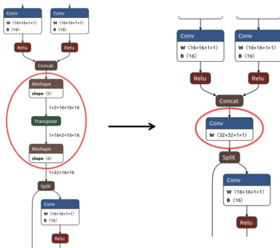
图8-7 卷积重排
