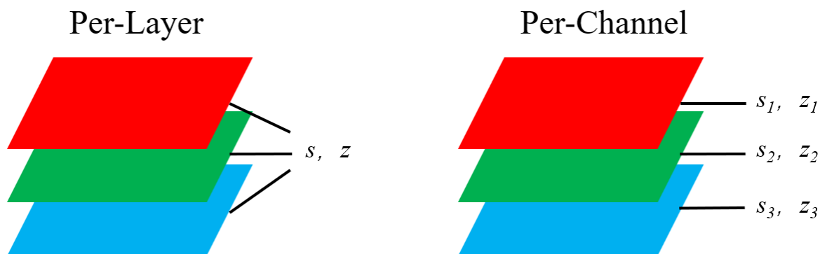
图6-2 Per-Layer量化和Per-Channel量化
