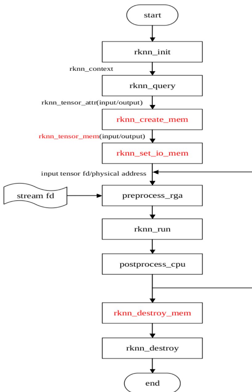
图5-7 零拷贝 API接口调用流程（输入/输出内部分配）
