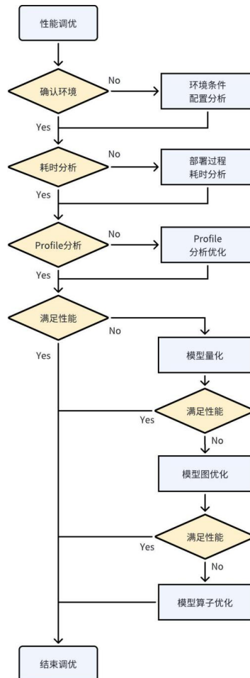
图8-1 模型性能优化流程
