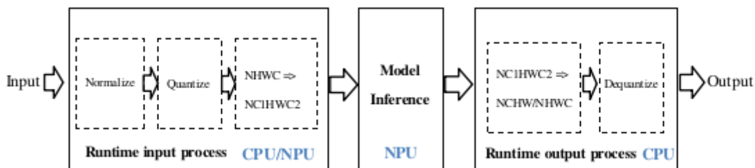
图5-5 通用API的数据处理流程
