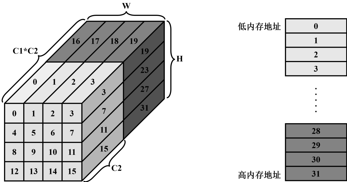
图5-1 RKNPU NC1HWC2数据排布与存储
