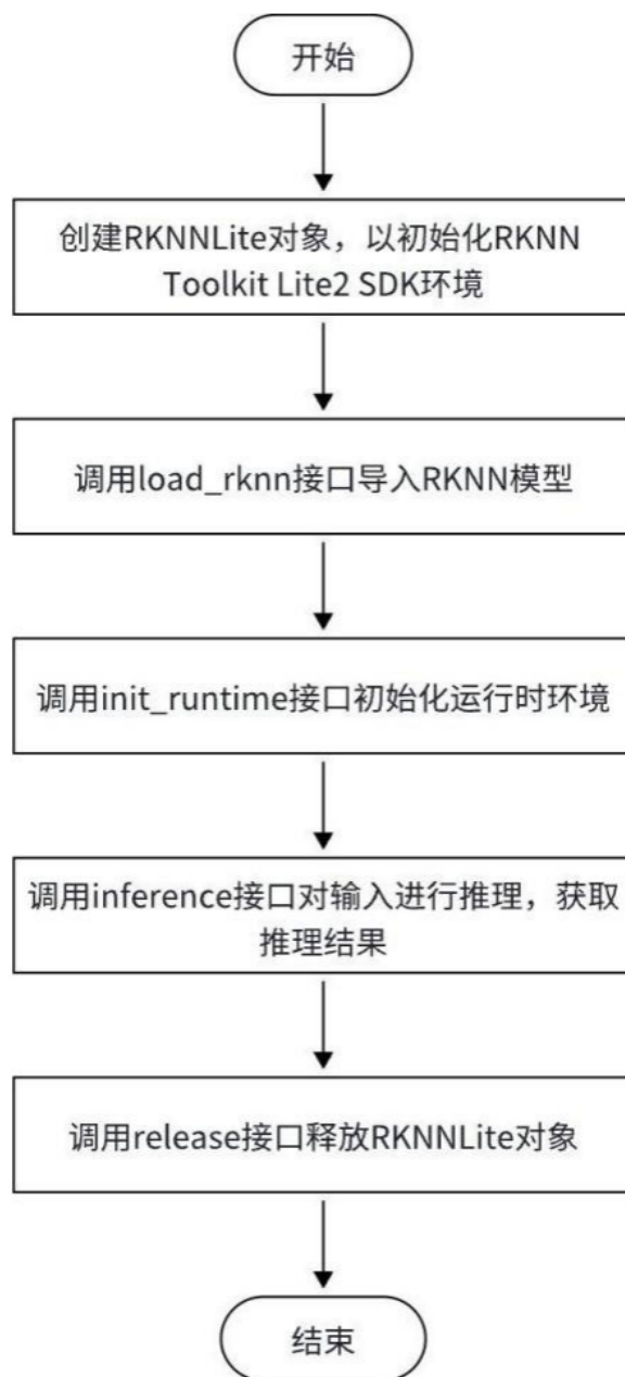
图3-5 RKNN-Toolkit Lite2基本使用流程
