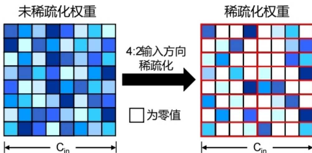
图5-16 4:2 输入方向稀疏化原理图
