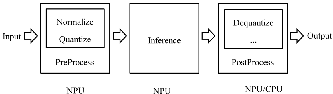
图1-4 零拷贝API数据处理流程
