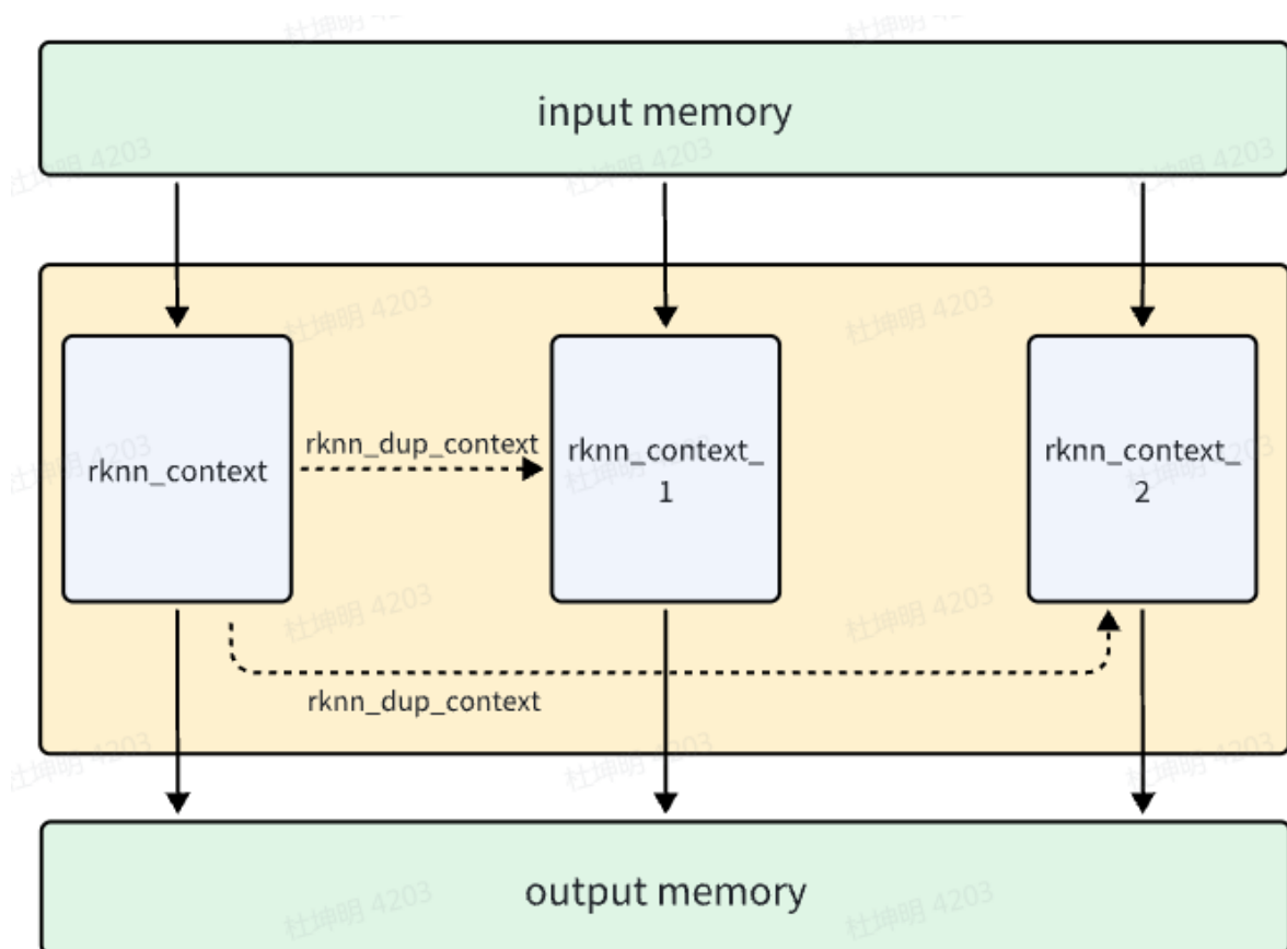
图5-14 多batch内部原理图
