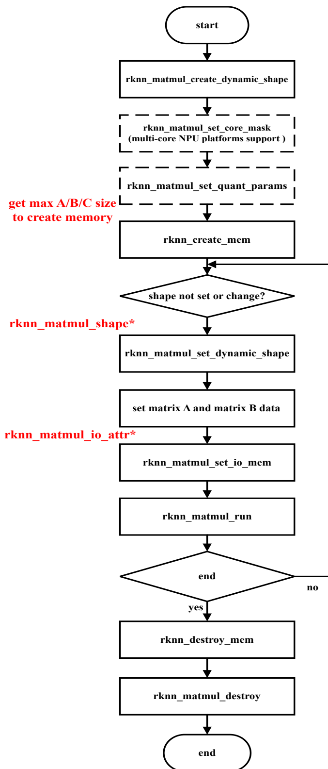
图3-7 动态shape输入的Matmul API调用流程
