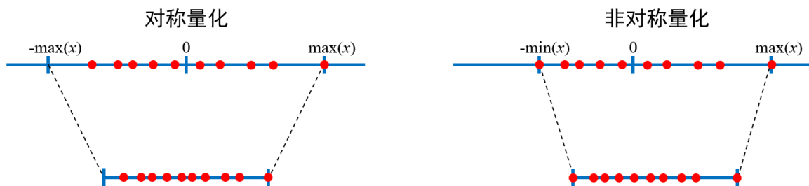
图6-1 线性对称量化和线性非对称量化
