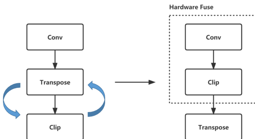
图8-8 算子图优化/融合
