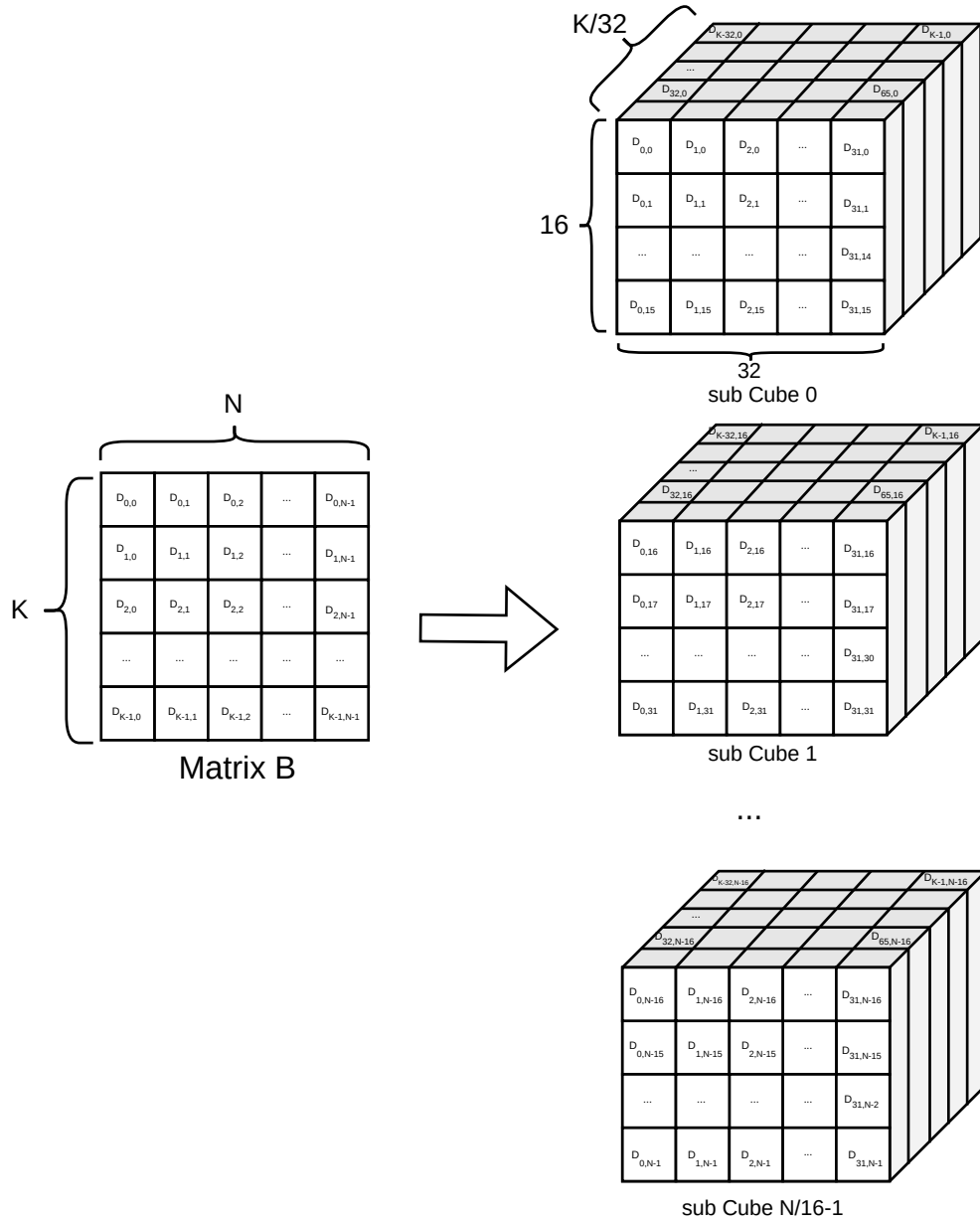
图3-9 int8类型矩阵B从[K,N]变换到[N/16,K/32,16,32]的元素对应关系图
