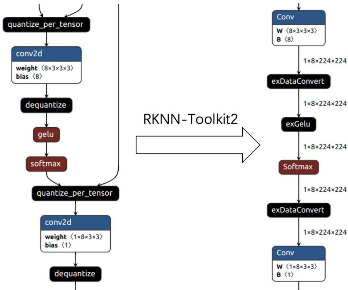
图6-6 QAT OP 前后为非量化算子状态
