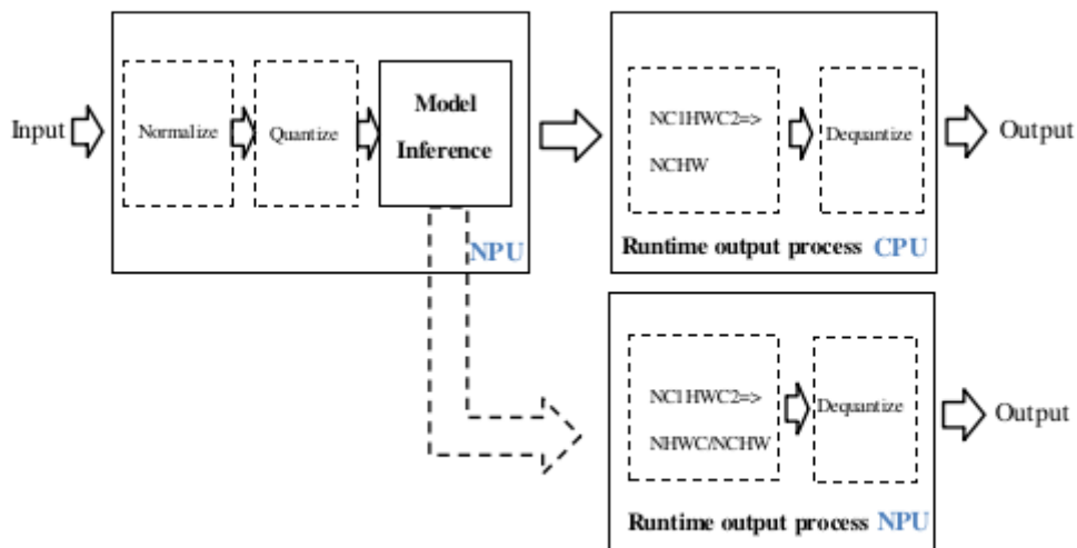
图5-6 零拷贝API数据处理流程
