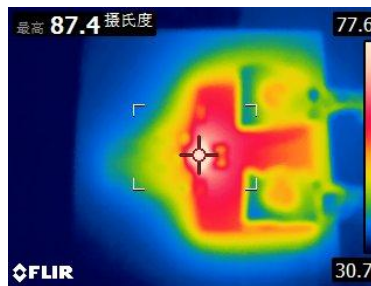
封装体热成像图（输入电流 35A）
