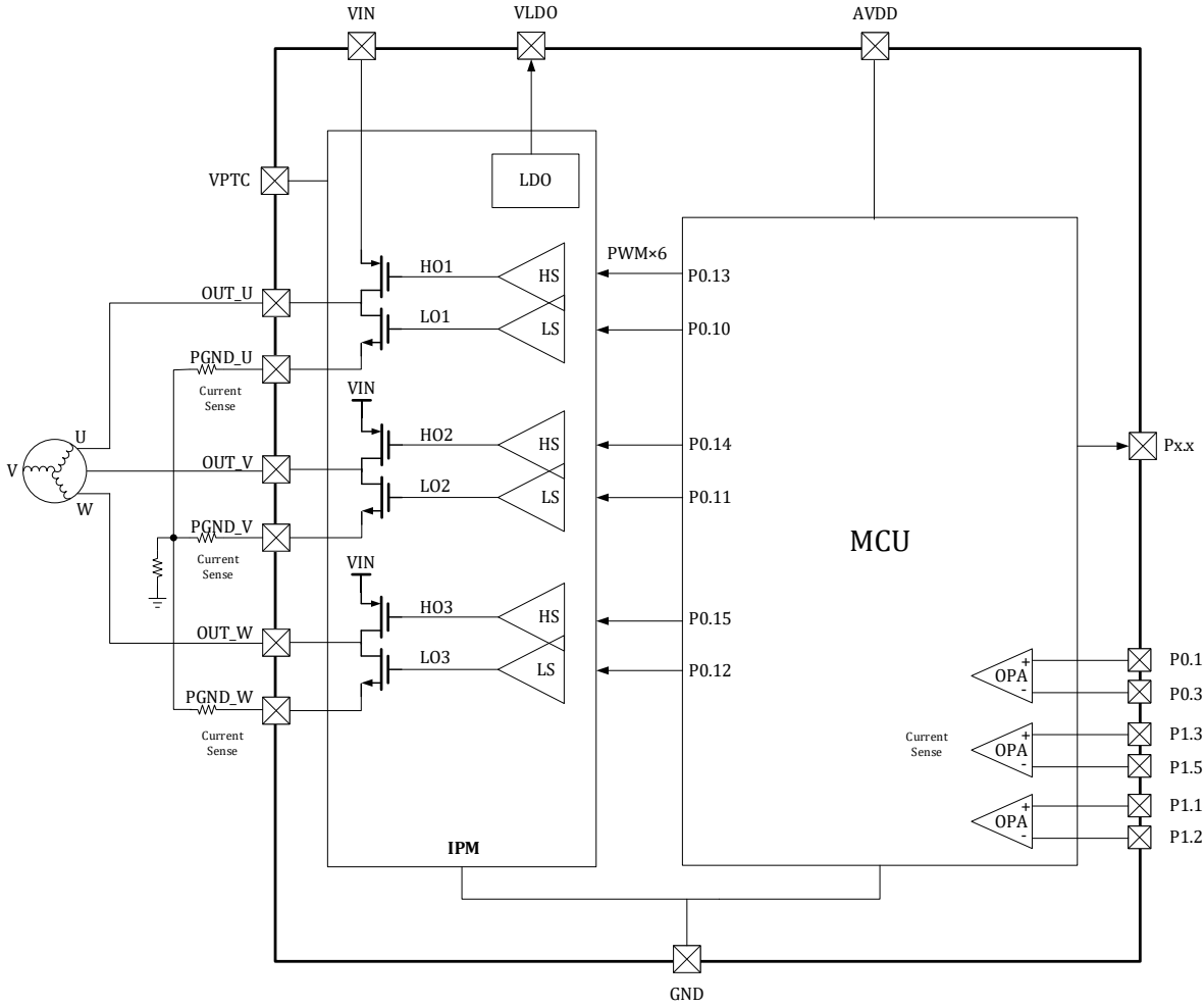
图 3-24 LKS32MC037QM6Q8 预驱连接示意图
