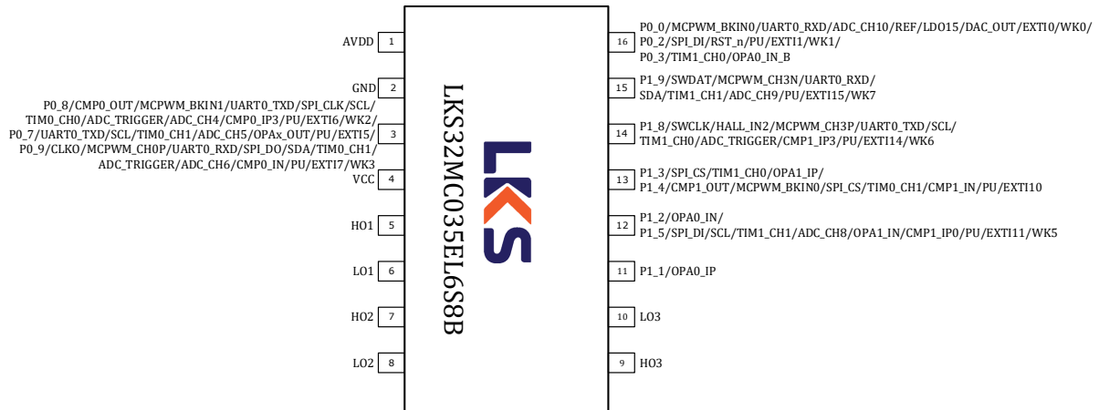
图 3-7 LKS32MC035EL6S8B(C)管脚分布图
