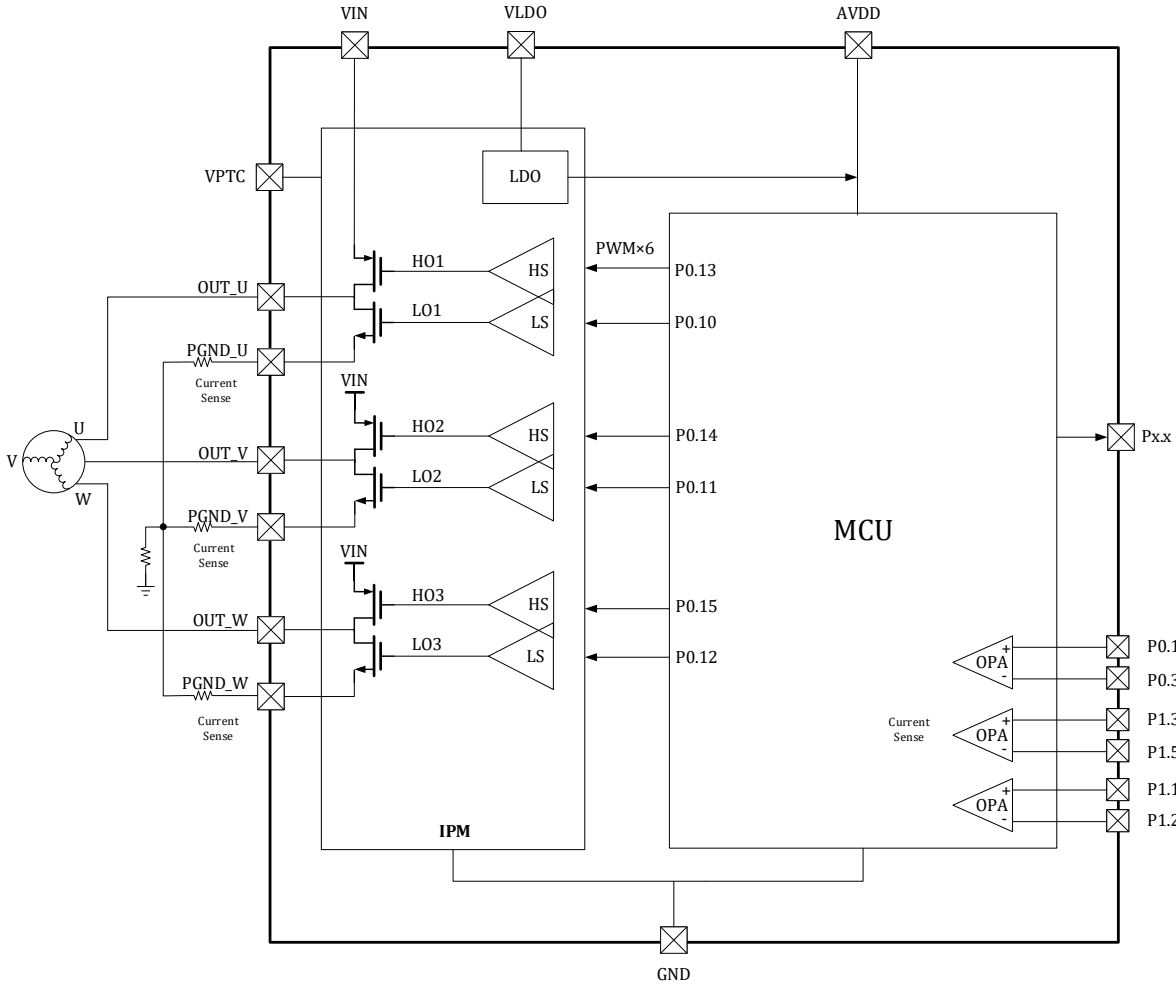
图 3-22 LKS32MC037QM6Q8 预驱连接示意图
