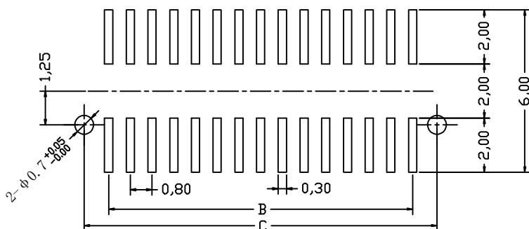
P.C.B PATTEN
