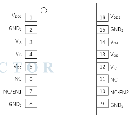
图 4.π131Mxx 管脚定义
