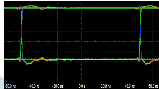
图 16. \pi 13xMxx 眼图
