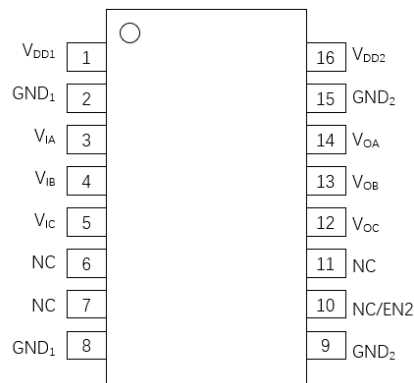
图 3.π130Mxx 管脚定义
