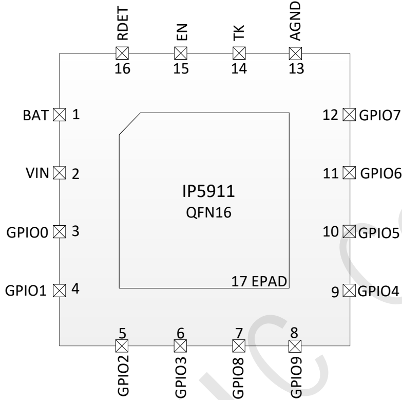
图 2 IP5911 引脚图
