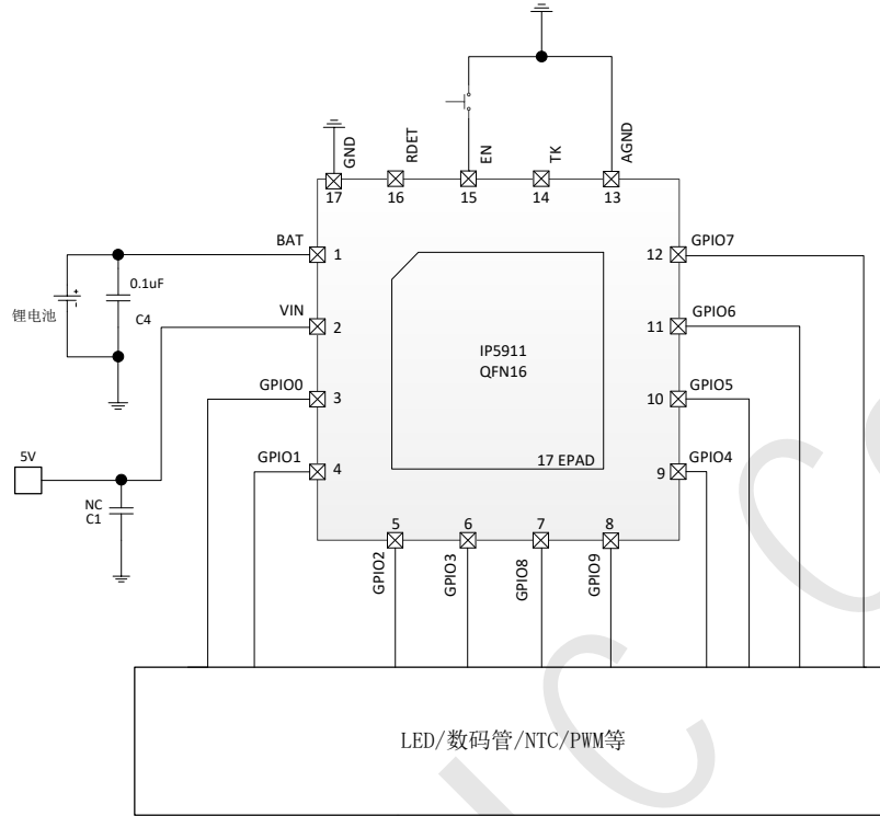
图 4 IP5911 典型应用原理图
