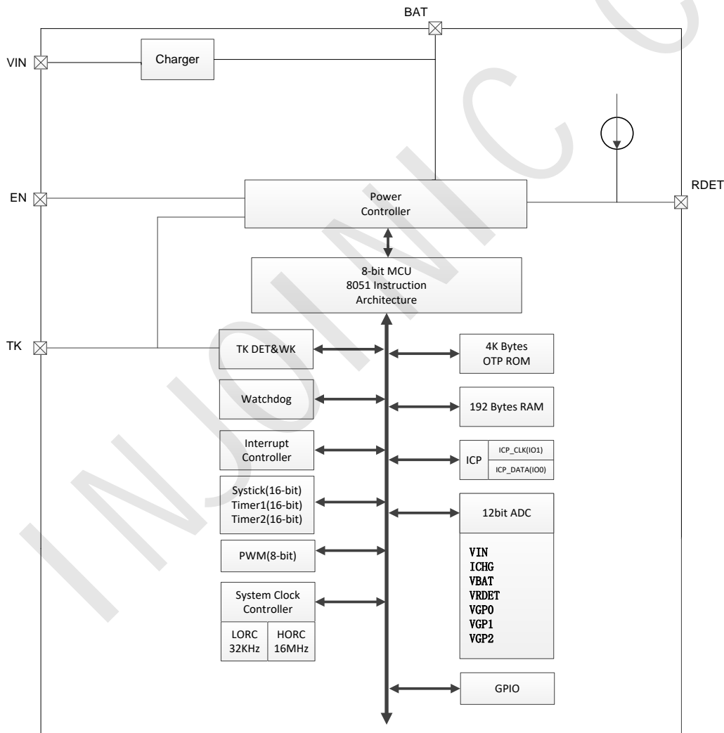
图 1 IP5911 内部系统框图
