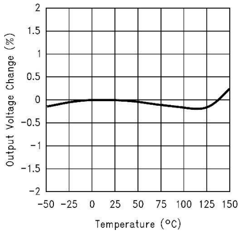
温度稳定性
