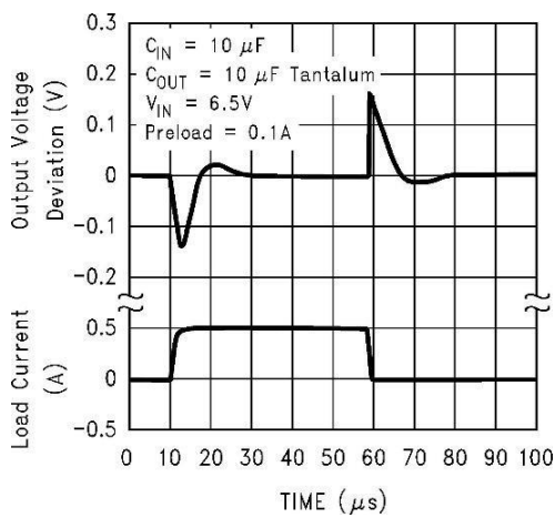
CBM1117X-5.0 线性瞬态响应
