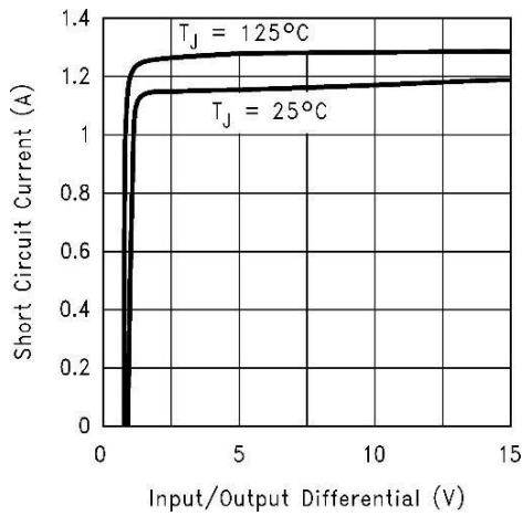
短路电流
