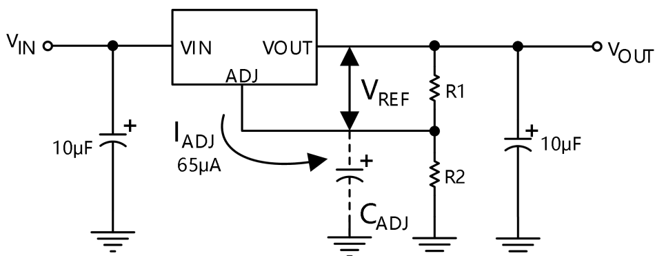
图 4. 基本可调调节器
