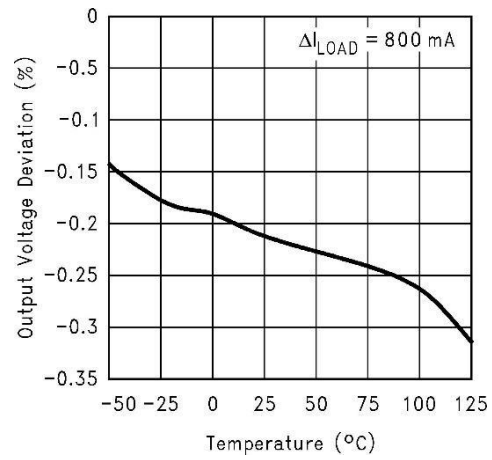
负载调整
