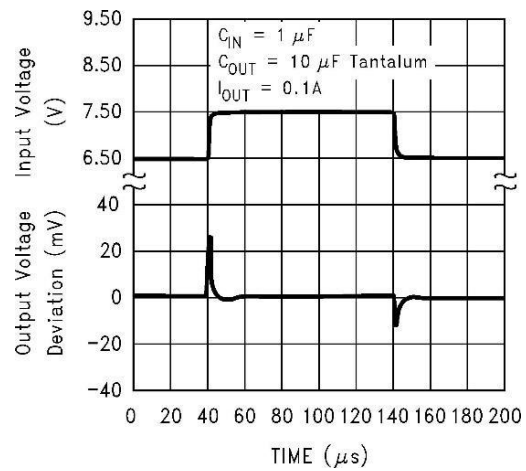
CBM1117X-5.0 线性瞬态响应
