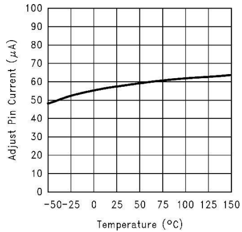
可调引脚电流
