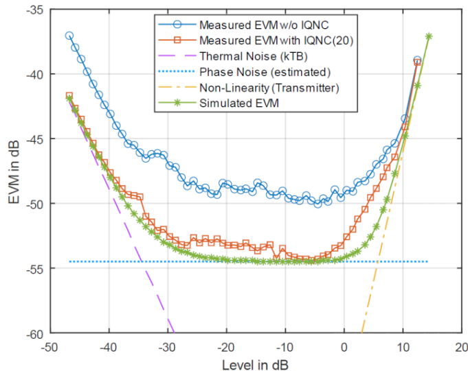
图11 IQ噪声抵消带来的EVM提升
