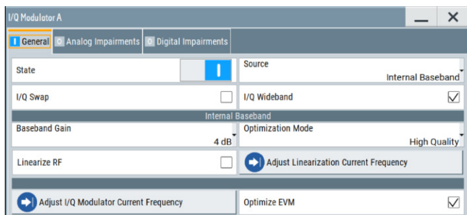
图3 信号源EVM优化功能
