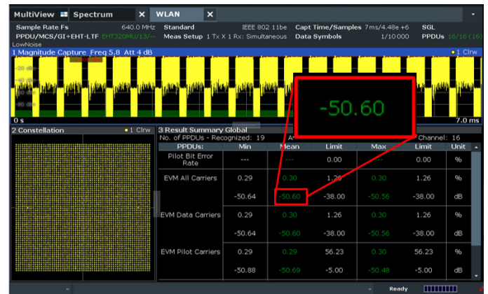
图2 Wi-Fi 7信号EVM测试结果
