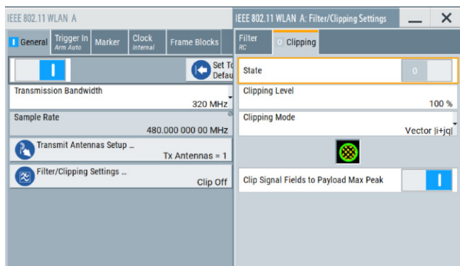
图4 信号源基带前导码削峰
