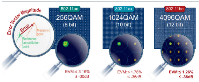
图1 越来越高的EVM要求
