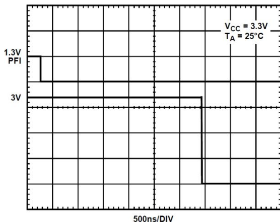
图 8.电源失效输入 (PFI) 低电平有效响应时间
