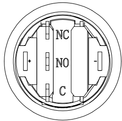
引脚图
