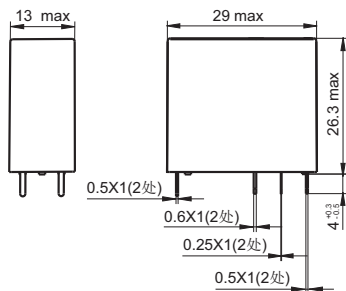
两组转换
