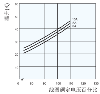
线圈温升
