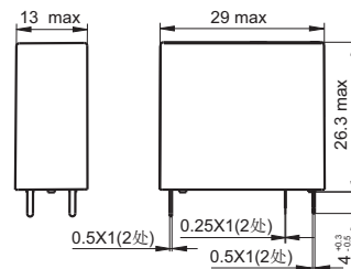
两组常开
