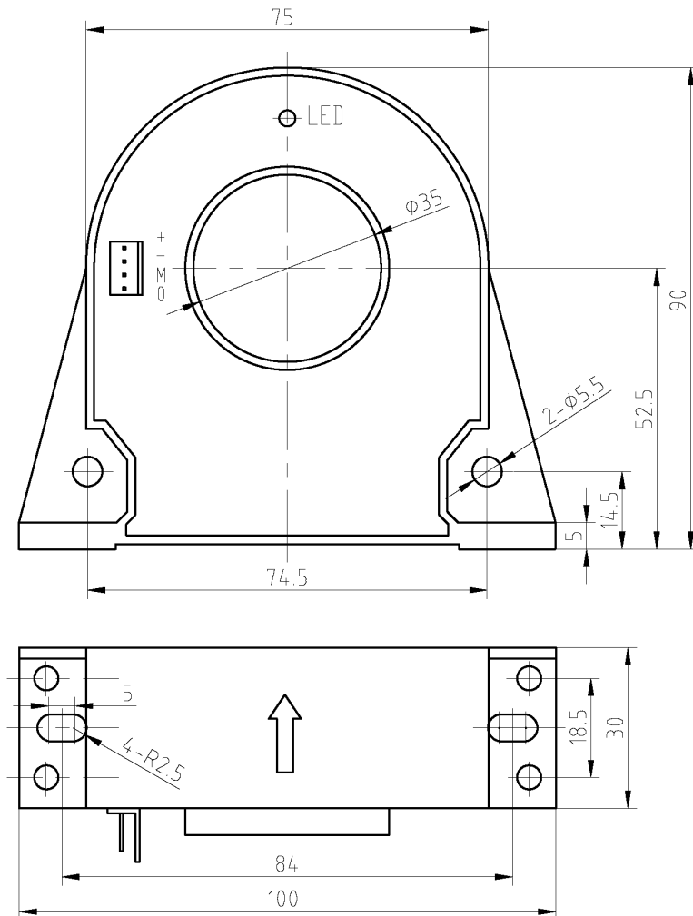
图 1 外形图
