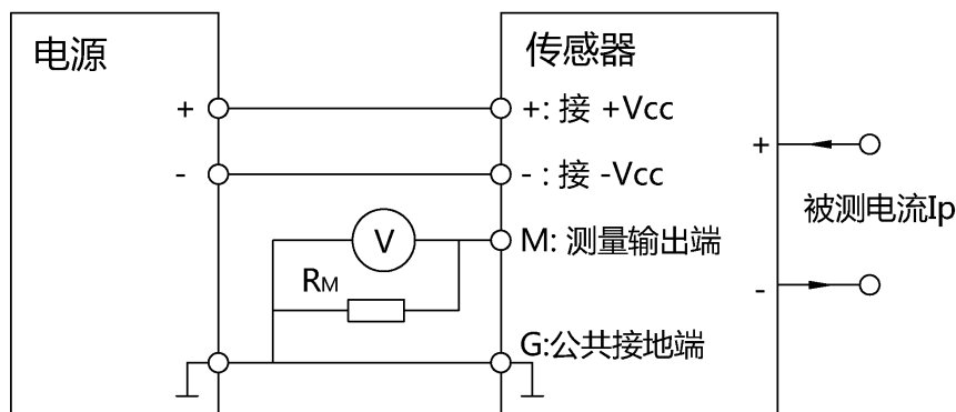
电气连接图
