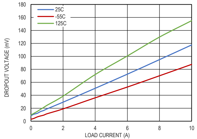
图 24. 最小输入电压和输出电压的关系, V_{OUT}=4.096V
