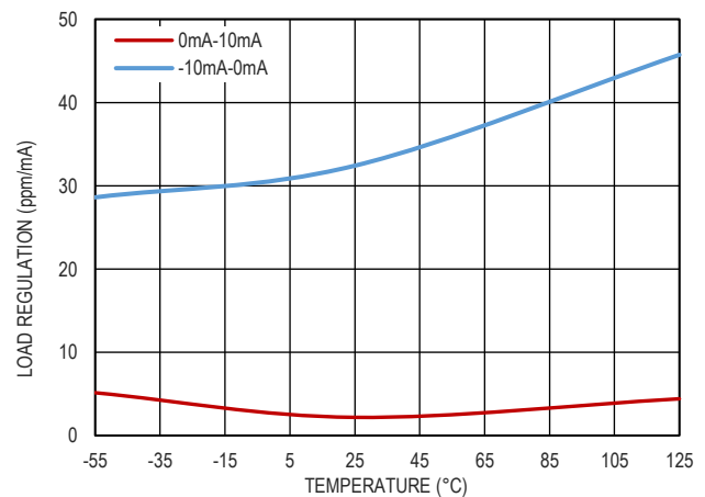
图 10. 负载调整率和温度的关系, V OUT =2.048V
