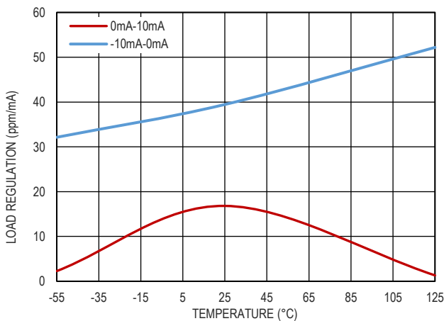
图 9. 负载调整率和温度的关系, V OUT =1.25V
