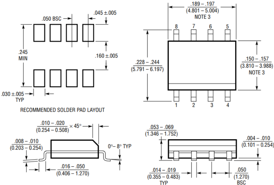
图 29.8 引脚 SO-8
