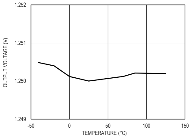
图 5. 1.25V 输出电压和温度的关系
