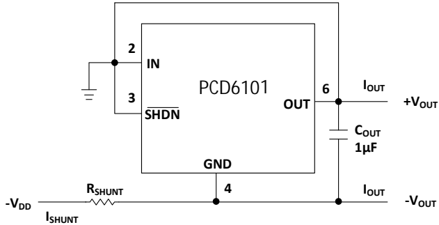
图 28. 负压并联方式
