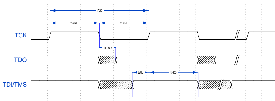
图 7: JTAG 时序图
