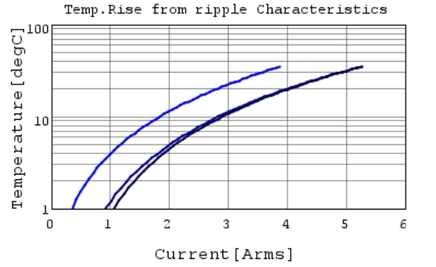
GRM219R60J106ME19 Temp.rise — 80kHz
