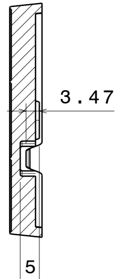
Section view B-B Scale: 1:1
