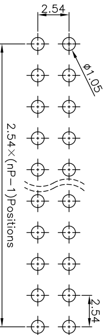
P.C.B LAYOUT
