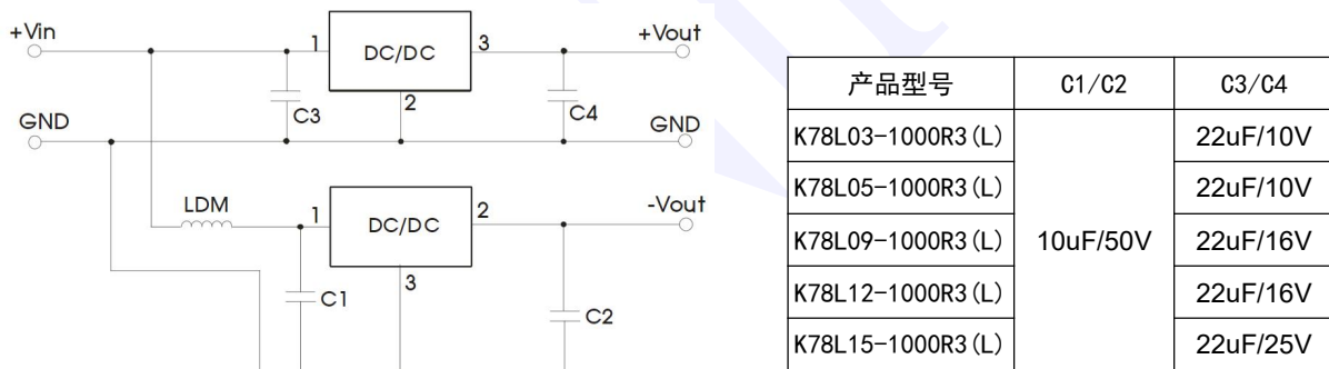
图 3 正负输出并联应用电路
