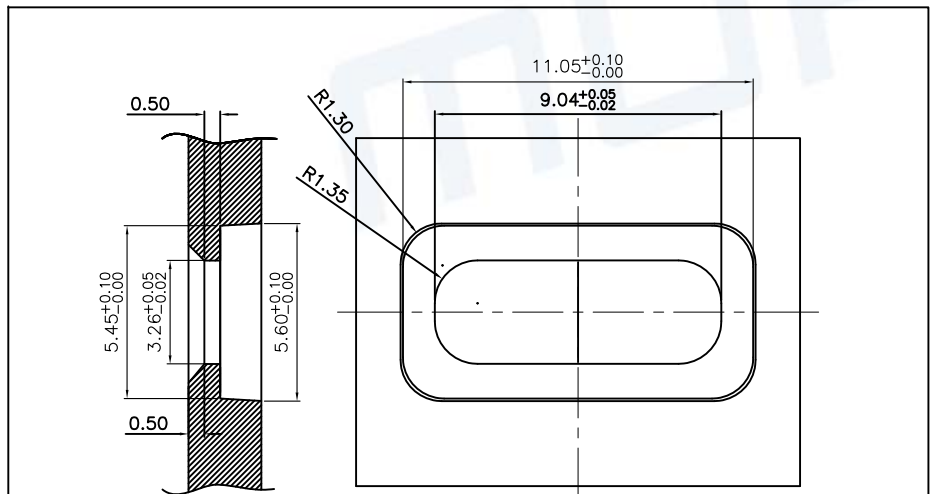
建议机壳面板设计尺寸 (以上尺寸仅供参考)
